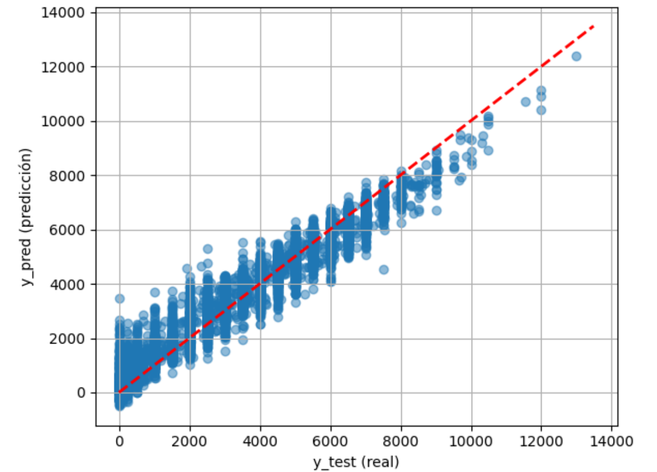
Predicción vs Realidad
