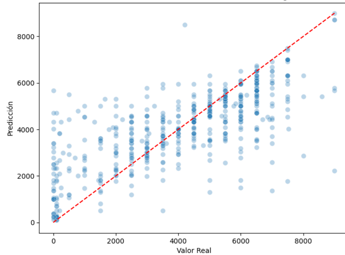
Scatter - Real vs Predicción (GradientBoosting)
